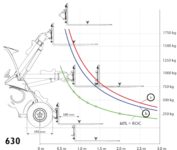
Diagrama de carga 630/635/640
